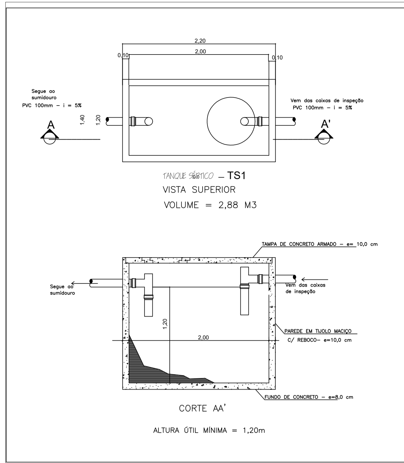
DETALHE DO TANQUE SÉPTICO
